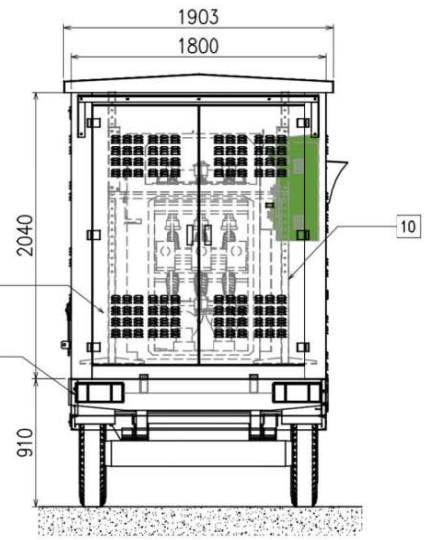
TAMPAK BELAKANG
